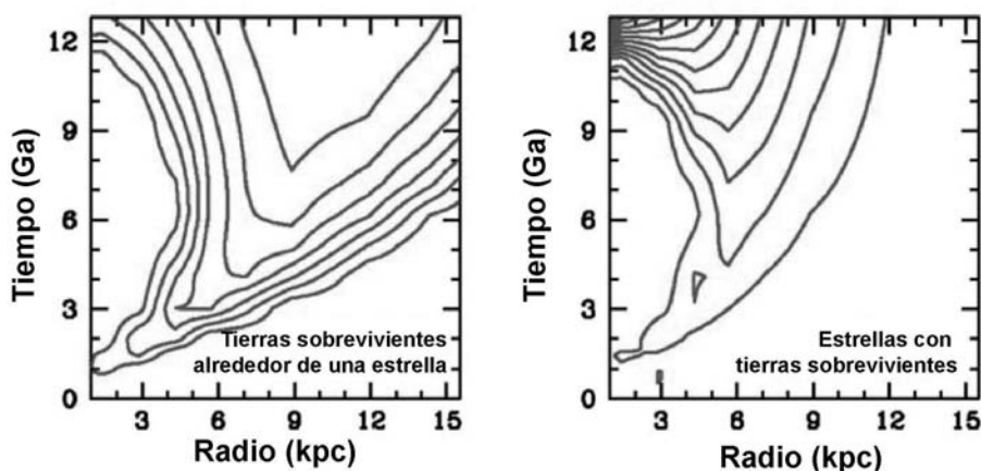
Fig. 3 - La GHZ según Prantzos (2006). A la izquierda se muestra las curvas de probabilidad de supervivencia para planetas de tipo terrestre. A la derecha, se convoluciona esta probabilidad con la densidad total de estrellas en la Galaxia, y por lo tanto se obtiene la densidad de estrellas con planetas habitables por seres vivos complejos (imagen cortesía Prof. Prantzos).
