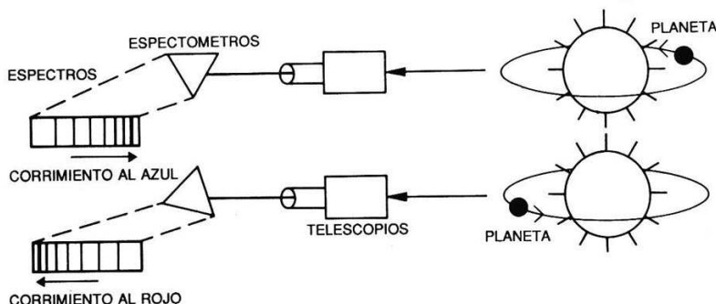
Fig. 2 - Corrimiento Doppler periódico de las líneas espectrales. Imagen reproducida con autorización de Lemarchand, (1992).
