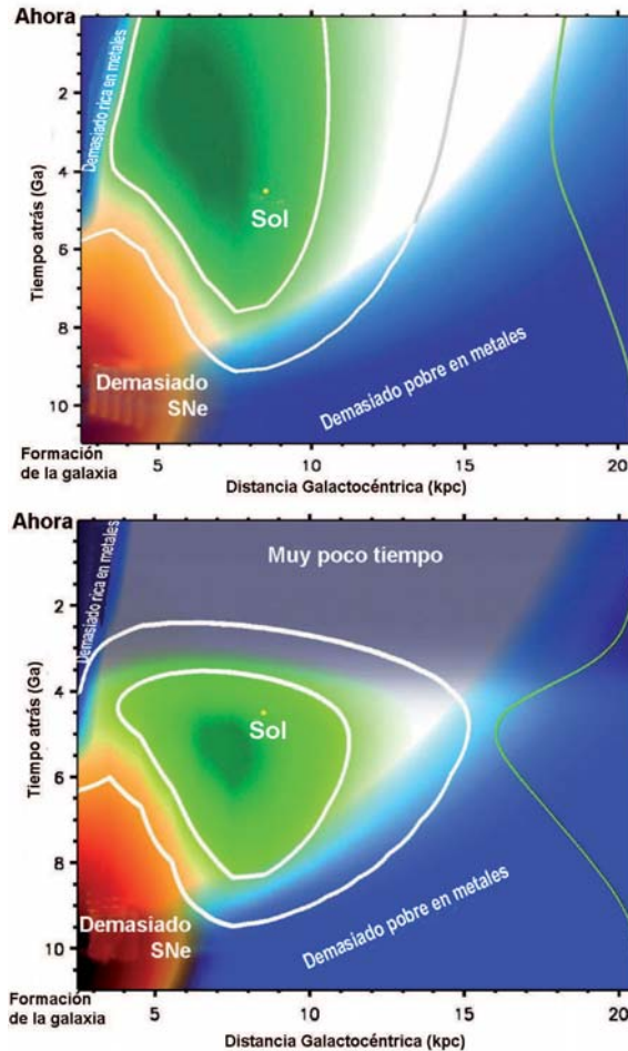
Fig. 2 - La zona habitable galáctica según Lineweaver et al., (2004). Las regiones habitables se encuentran rodeadas por curvas blancas. En la figura de arriba se exige una media de 4.000 millones de años para la aparición de vida compleja, mientras que en la de abajo se elimina dicha restricción (imágenes cortesía del Prof. Lineweaver).
