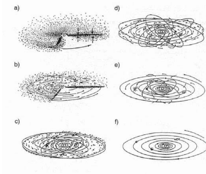
Fig. 1 - Proceso de formación del Sistema Solar. Cortesía Gonzalo Tancredi
