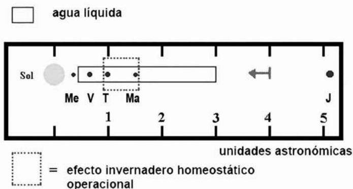
Fig. 4 – Límites de la zona de habitabilidad en el Sistema Solar. El cuadro con línea continua simplemente muestra los límites donde el agua líquida podría existir por simples efectos de temperatura. El cuadro punteado muestra los límites actuales de la zona de habitabilidad, por la restricción “pesimista” del texto.
