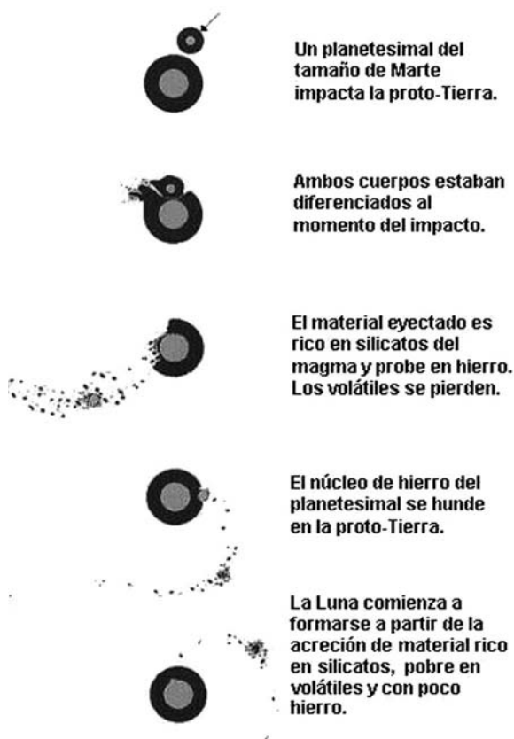
Fig. 6 - Esquema de la formación del sistema Tierra-Luna a partir de la colisión de un planetesimal del tamaño de Marte con la proto-Tierra.
