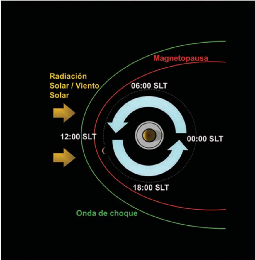
Fig. 1 - Esquema que representa la magnetósfera de Saturno (región dentro de la curva roja, la magnetopausa) y Titán, que en órbita a 20 radios planetarios, se enfrenta al plasma de la magnetósfera que rota con el planeta (flechas celestes). La dirección del plasma incidente y la de los fotones solares (flechas doradas) va variando a lo largo de la órbita y es función del tiempo local de saturno (SLT). Así, las dos direcciones son antiparalelas a 06:00 SLT y paralelas a 18:00 SLT.
