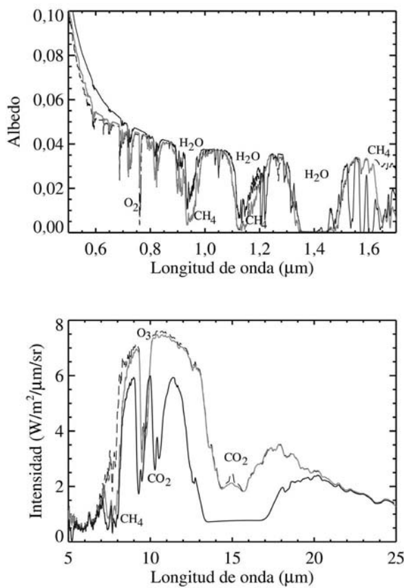
Fig. 3 - Espectro terrestre en tres diferentes etapas: Arqueano (línea negra continua), Proterozoico medio (línea gris) y Presente (línea discontinua) ( Fuente: Segura et al. 2003, 2005 y 2007).
