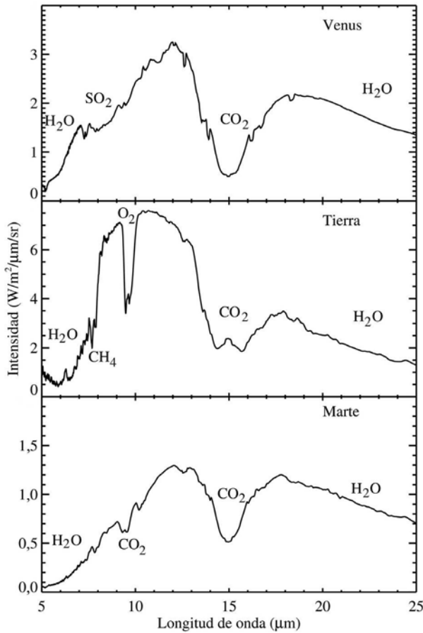
Fig. 2 - Espectros sintéticos de Venus, Tierra y Marte en el infrarrojo medio generados por el Virtual Planetary Laboratory (VPL) ( Fuente: V.S. Meadows, U. Washington).
