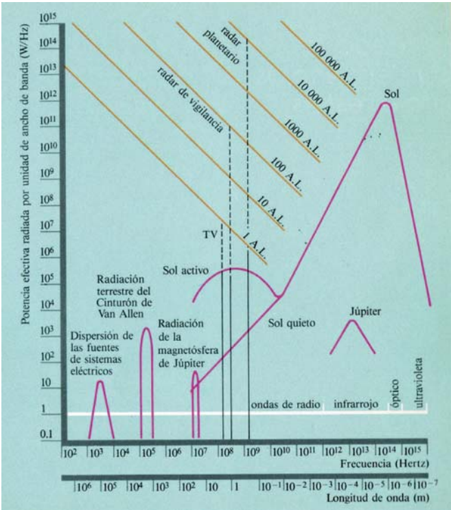
Fig. 1 - Diagrama indicativo de las potencias efectivas radiadas por diversas fuentes del sistema solar, expresadas en Watts por unidad de ancho de banda en función de la frecuencia y de la longitud de onda. Fuente: Colomb y Lemarchand (1989).
