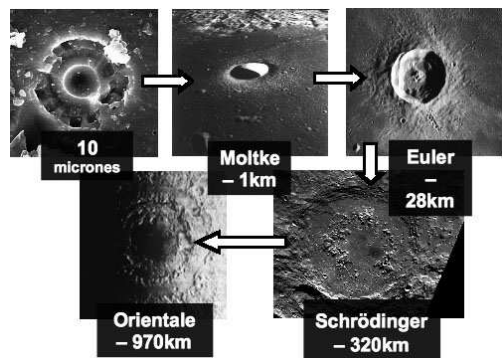
Fig. 2 - Secuencia de estructuras de impacto
