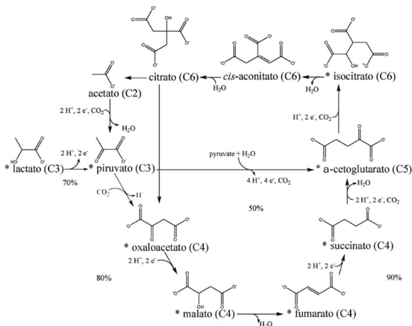
Fig. 7 - Moléculas del CIATC generadas en reacciones fotoquímicas sobre ZnS.
