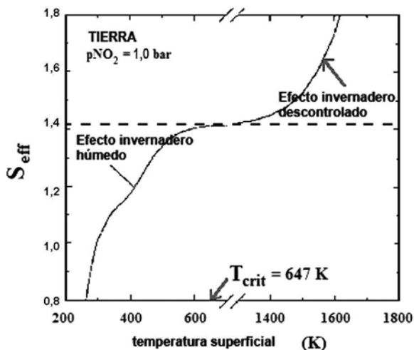
Fig. 3 – Los límites físicos internos de la zona de habitabilidad, el efecto invernadero húmedo, y el efecto invernadero descontrolado. En el primero se obtiene S_{\text{eff}} = 1,10 , y en el segundo S_{\text{eff}} = 1,41 .
