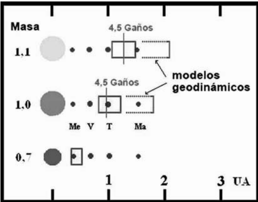
Fig. 5 – Zona de habitabilidad continua para diversas masas estelares, basadas en los límites “pesimistas” discutidas en el texto. Los cuadros continuos señalan los límites actuales. Modelos geodinámicos permiten una extensión de los límites externos a distancias más grandes en las fases iniciales de evolución estelar.
