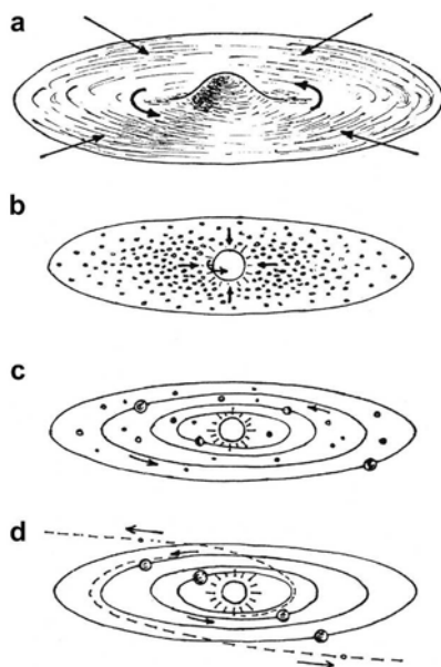
Fig. 3 - Las distintas etapas de la formación del Sistema Solar y la dispersión del material residual: (a) Colapso gravitacional de la nube de gas y polvo en el protosol y el disco protoplanetario; (b) formación en el disco de planetesimales de tamaño típico de algunos km; (c) acumulación de planetesimales en un número reducido de embriones planetarios; (d) crecimiento oligárquico en unos pocos planetas masivos y dispersión de los planetesimales residuales por interacciones gravitacionales con los planetas formados (Fernández 2005).
