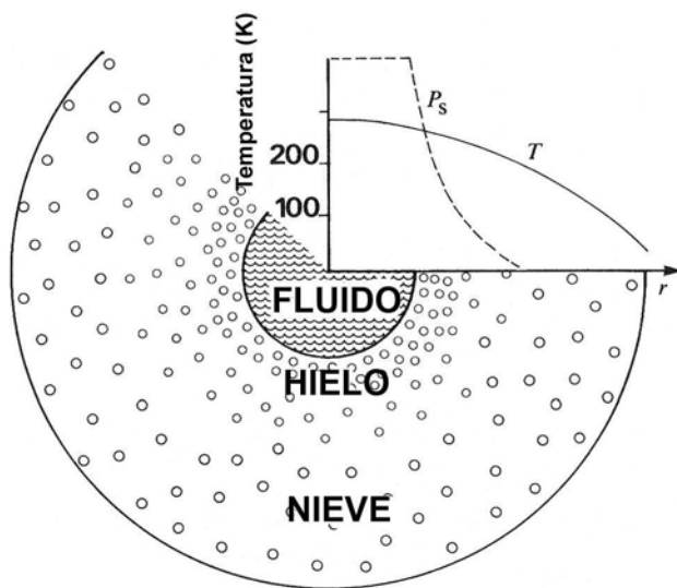
Fig. 10 - Hipotético núcleo de agua líquida de un núcleo cometario. Se grafican también la presión de vapor P_s y la temperatura T computadas en función de la distancia r al centro (Wallis 1980).
