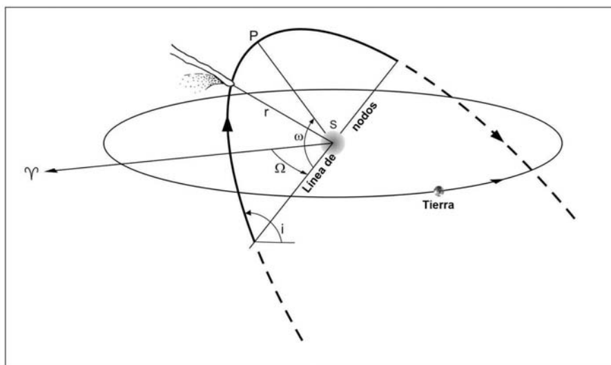
Fig. 5 - Elementos orbitales (tomado de Fernández 2005).
