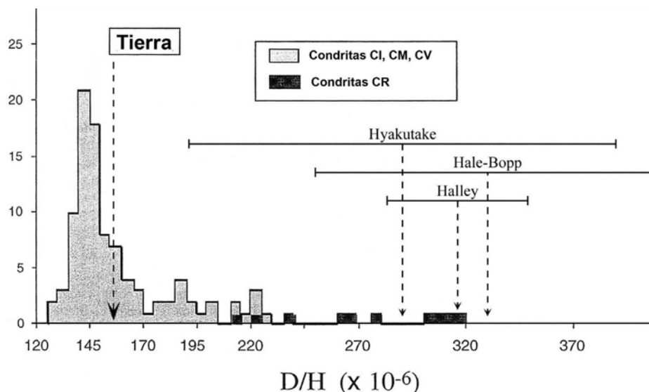
Fig. 9 - Distribución del cociente de isótopos D/H en una muestra de meteoritos del tipo de las condritas carbonosas (tomado de Robert 2003). Se indican también los valores correspondientes al agua oceánica y los valores medidos en los cometas 1P/Halley, C/1995 O1 (Hale-Bopp) y C/1996 B2 (Hyakutake) (Fernández 2005).
