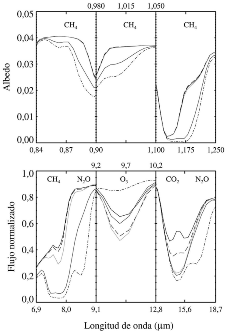
Fig. 6 - Bandas prominentes de CH 4 , N 2 O, O 3 , y CO 2 en espectros de planetas como la Tierra alrededor de estrellas F, G, K y M con las resoluciones planeadas para TPF y Darwin: 70 para el visible e infrarrojo cercano (panel superior) y 25 para el infrarrojo medio (panel inferior). El espectro en el infrarrojo medio está normalizado a un cuerpo negro con temperatura de 288 K. Clave: planeta alrededor de la estrella F: línea negra continua; planeta alrededor de la estrella G: línea negra discontinua; planeta alrededor de la estrella K: línea gris claro; planeta alrededor de la estrella M (AD Leo): línea gris oscuro; planeta alrededor de la estrella M(3100K): punto-rama negra. ( Fuente: Segura et al. 2003 y 2005).
