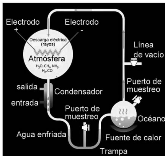
Fig. 2 - El experimento de Miller.
