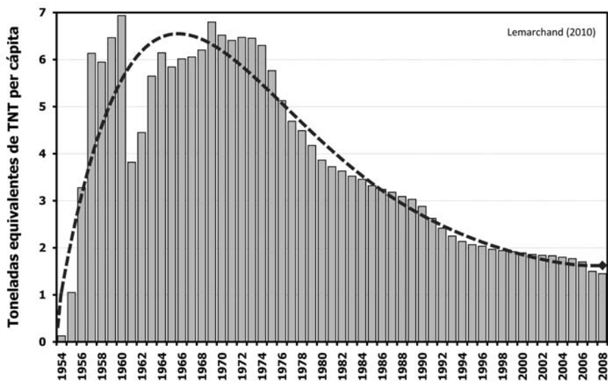
Fig. 7 - Evolución de la capacidad destructiva equivalente del armamento nuclear desplegado por año dividido el valor la población mundial anual (1954-2008). Fuente: Lemarchand (2010).
