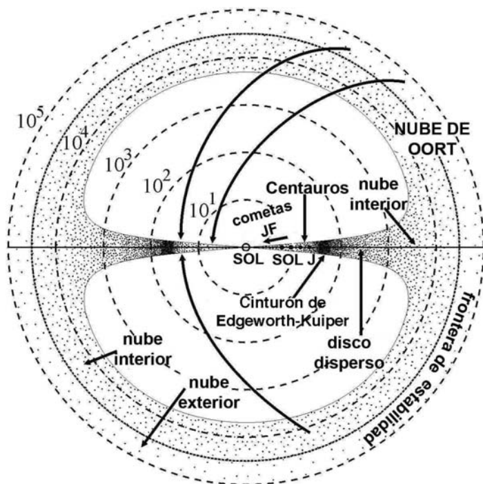
Fig. 7 - Esquema que muestra la distribución de las diferentes poblaciones de objetos ricos en hielos del Sistema Solar, yendo desde los cometas de la Familia de Júpiter, Centauros, objetos transneptunianos, hasta la nube de Oort. Las flechas curvadas representan la vía de ingreso a la región planetaria de cometas de la nube de Oort. Los círculos concéntricos punteados indican distancias en UA (Fernández 2005).
