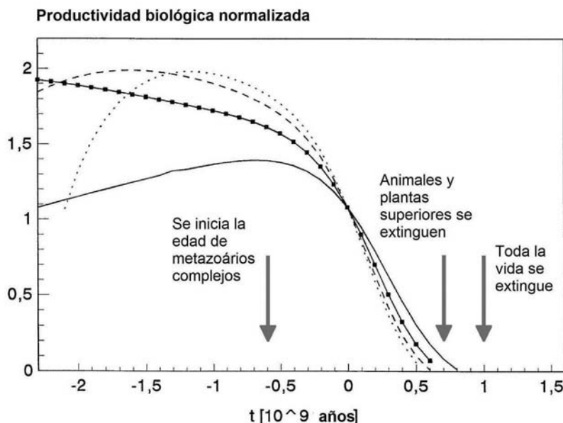
Fig. 8 – El límite temporal de habitabilidad de la Tierra medido por la bioproductividad. La necesidad de disminuir la concentración de dióxido de carbono en la Tierra para mantener la temperatura hará imposible el proceso de fotosíntesis en el futuro, terminando con la biosfera.
