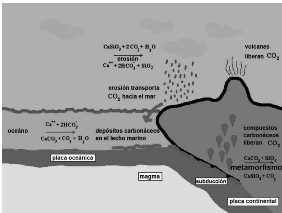
Fig. 1 – Ilustración del mecanismo del ciclo carbonato-silicato de actuación para el mantenimiento de la temperatura superficial de la Tierra dentro de los límites de existencia de agua líquida
