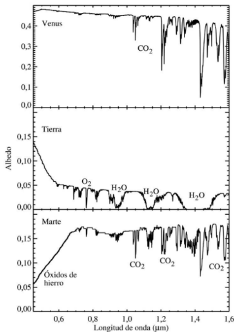
Fig. 1 - Espectros sintéticos de Venus, Tierra y Marte en el visible e infrarrojo cercano generados por el Virtual Planetary Laboratory (VPL) (Fuente: V.S. Meadows, U. Washington).
