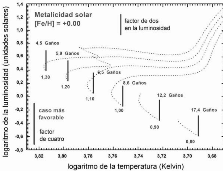
Fig. 7 – Tiempos de vida para estrellas de distintas masas y metalicidad solar. Las luminosidades iniciales están en los puntos de partida de las trayectorias evolutivas (en masas solares: líneas discontinuas). En las abscisas se muestra el logaritmo de la temperatura, en las ordenadas, el de la luminosidad. Las barras corresponden a un aumento de luminosidad de un factor dos (caso pesimista discutido en el texto), la barra contra el eje izquierdo inferior indica un factor cuatro (caso optimista). Las edades para llegar a un factor dos de aumento de luminosidad desde la edad cero están señaladas al lado de las trayectorias.
