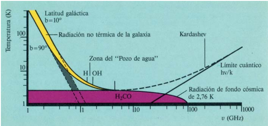
Fig. 2 - Intensidad de ruido de las fuentes naturales de radiación (expresadas en grados Kelvin) en función de la frecuencia. Se representan algunos ejemplos de “frecuencias mágicas” sugeridas para la comunicación interestelar. Fuente: Colomb y Lemarchand (1989).
