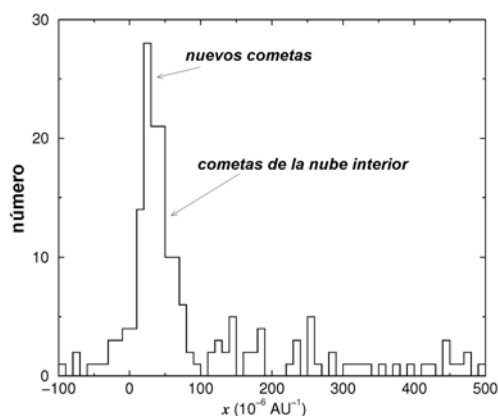
Fig. 6 - Distribución de las energías orbitales de cometas de largo período con energías x < 500 \times 10^{-6} \text{ UA}^{-1} (semiejes mayores a > 2000 \text{ UA} ). La muestra de cometas fue extraída del catálogo de Marsden & Williams (2008).
