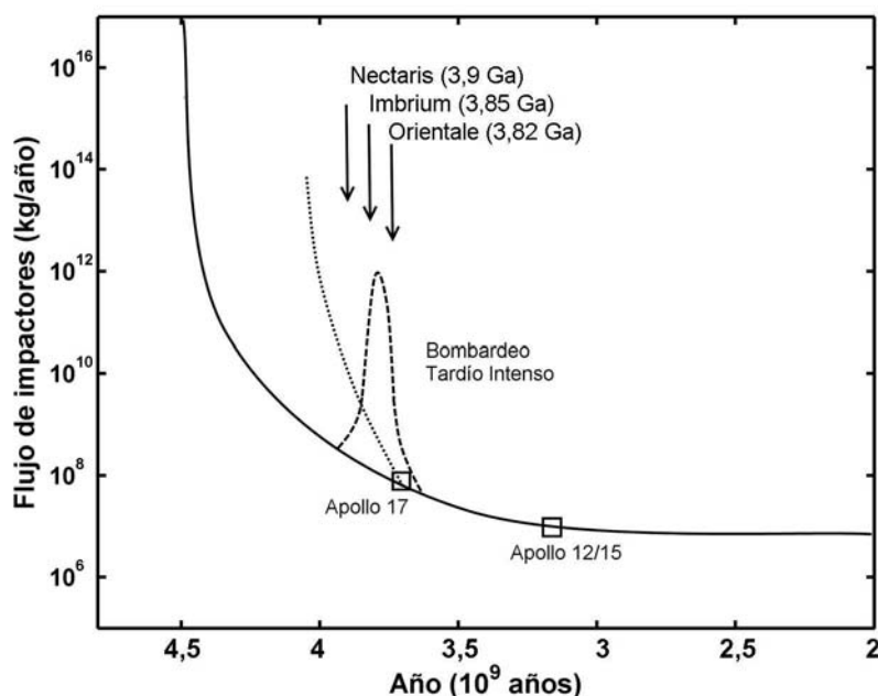
Fig. 8 - Tasa de impacto en la Tierra. La línea llena representa un decaimiento exponencial en el flujo de impactores, y la trayectoria punteada representa el incremento temporal ocurrido durante el LHB. Las edades de las principales cuencas de impacto de la Luna están indicadas (adaptado de Koebert, 2003 y de Tajika, 2008).
