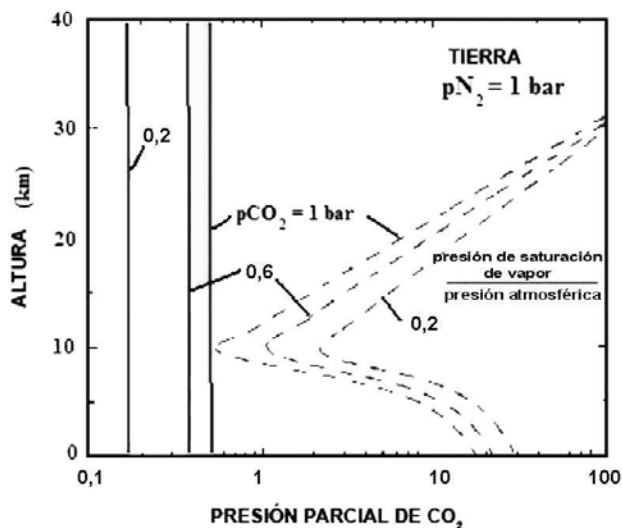
Fig. 2 – El límite físico de la zona de habitabilidad fijado por la primera formación de nubes de CO 2 . En las abscisas, la presión parcial de CO 2 en la atmósfera, en las ordenadas, la altitud. El aumento de la concentración de CO 2 provoca la condensación a una presión de un bar, cuando la presión atmosférica equivale a la presión de saturación.
