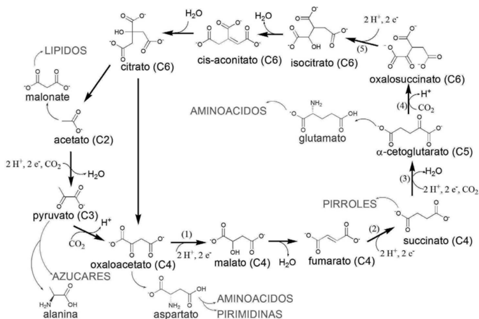
Fig. 4 - El ciclo inverso de los ácidos tricarboxílicos (CIATC), eje central del metabolismo universal.
