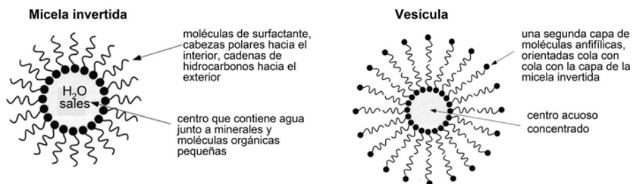
Fig. 3 - Orientación de los ácidos grasos en una micela invertida y en una vesícula.
