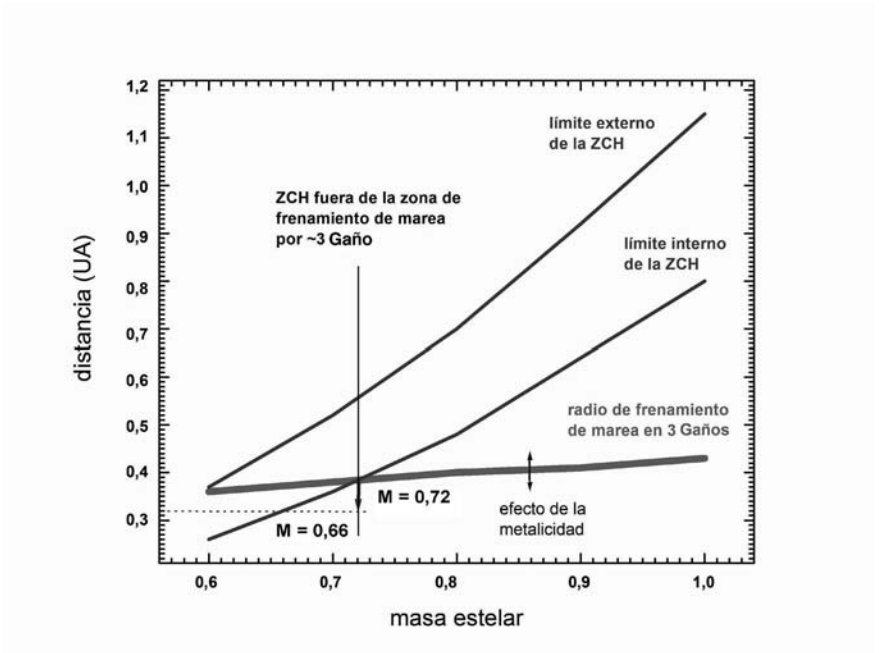
Fig. 6 – Zonas de frenado de marea para un tiempo de 3000 millones de años, para estrellas de metalicidad solar y distintas masas. Estrellas de masa superior a 0,7 masas solares tienen su zona de habitabilidad libre de problemas de frenado por alrededor de 3000 millones de años. El efecto de cambiar la metalicidad (y por consecuencia la luminosidad) de la estrella por un factor dos está ilustrado.
