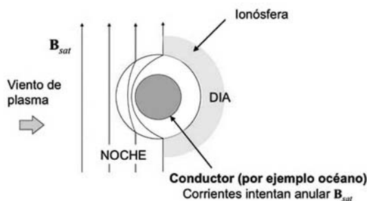
Fig. 3 - Esquema que describe la geometría de la interacción entre el campo magnético de Saturno y Titán a 06:00 horas de tiempo local (SLT). En este sector de la órbita de Titán, el plasma magnetosférico que transporta el campo magnético del planeta incide en el hemisferio nocturno, donde la ausencia de ionósfera (en amarillo) permite que B_{sat} llegue a la superficie y sea capaz de generar un campo inducido si existe un conductor en su interior.
