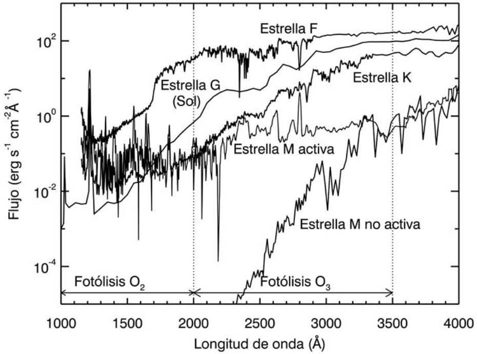
Fig. 4 - Radiación ultravioleta que recibe un planeta en la zona habitable de una estrella tipo F, una estrella G, una estrella M activa y una estrella M no activa ( Fuente M. Cohen, U. California, Berkeley).
