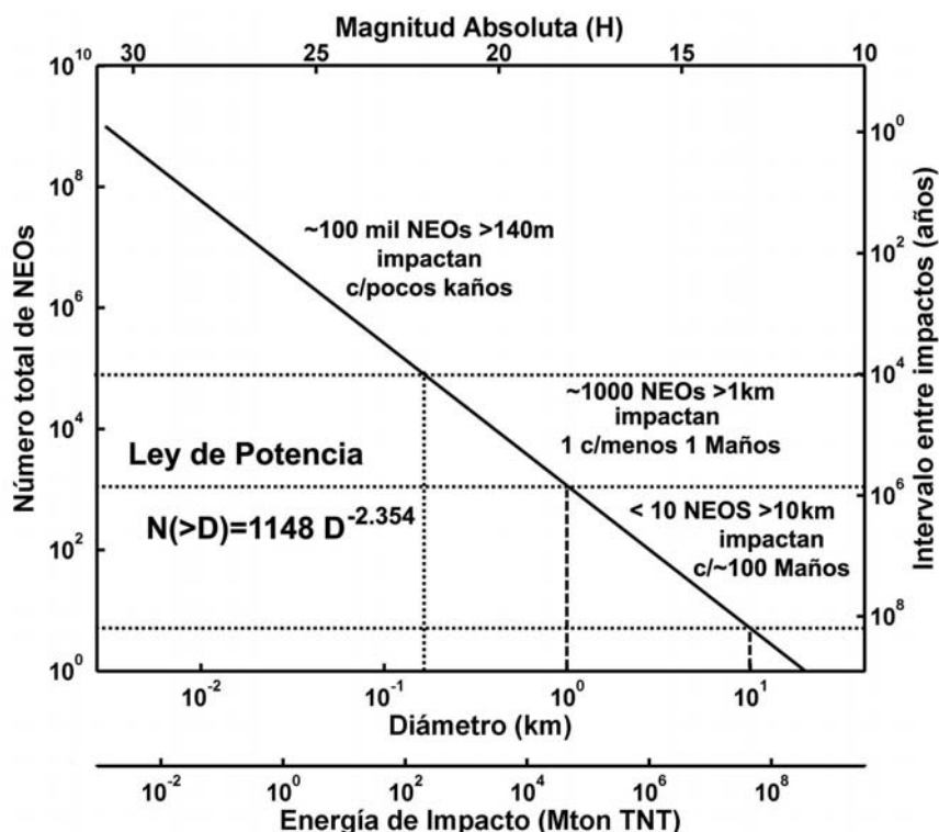
Fig. 15 - Distribución acumulativa de NEAs en función de diversos parámetros como: magnitud absoluta, tamaño o energía de impacto. Se considera una ley potencial como buen ajuste a los datos observados (NASA's NEO Report, 2007). También se muestra la frecuencia de impacto y la comparación con alguno de los eventos de impacto.
