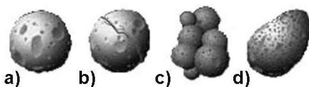
Fig. 5 - Modelos de estructura interna de asteroides: a) Sólido con cráteres superficiales; b) Sólido con grandes fracturas internas; c) Pila de escombros cubierta por polvo; d) Aglomerado de pequeñas rocas.
