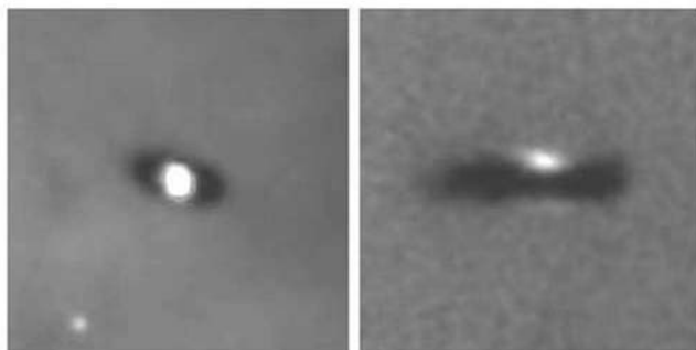
Fig. 2 - Imágenes del Telescopio Espacial Hubble de 2 discos protoplanetarios en la nebulosa de Orión iluminados en sus zonas centrales por la luz proveniente de sus estrellas jóvenes (McCaughrean & O'Dell 1996).
