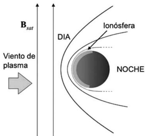
Fig. 2 - Esquema que describe la geometría de la interacción entre el campo magnético de Saturno y Titán a 18:00 horas de tiempo local (SLT). En este sector de la órbita de Titán, el plasma magnetosférico que transporta el campo magnético del planeta incide en el hemisferio diurno, donde la ionósfera (en amarillo) impide que B_{sat} llegue a la superficie. En esta configuración se mide el campo intrínseco de Titan, B_{int} , si es que posee uno.
