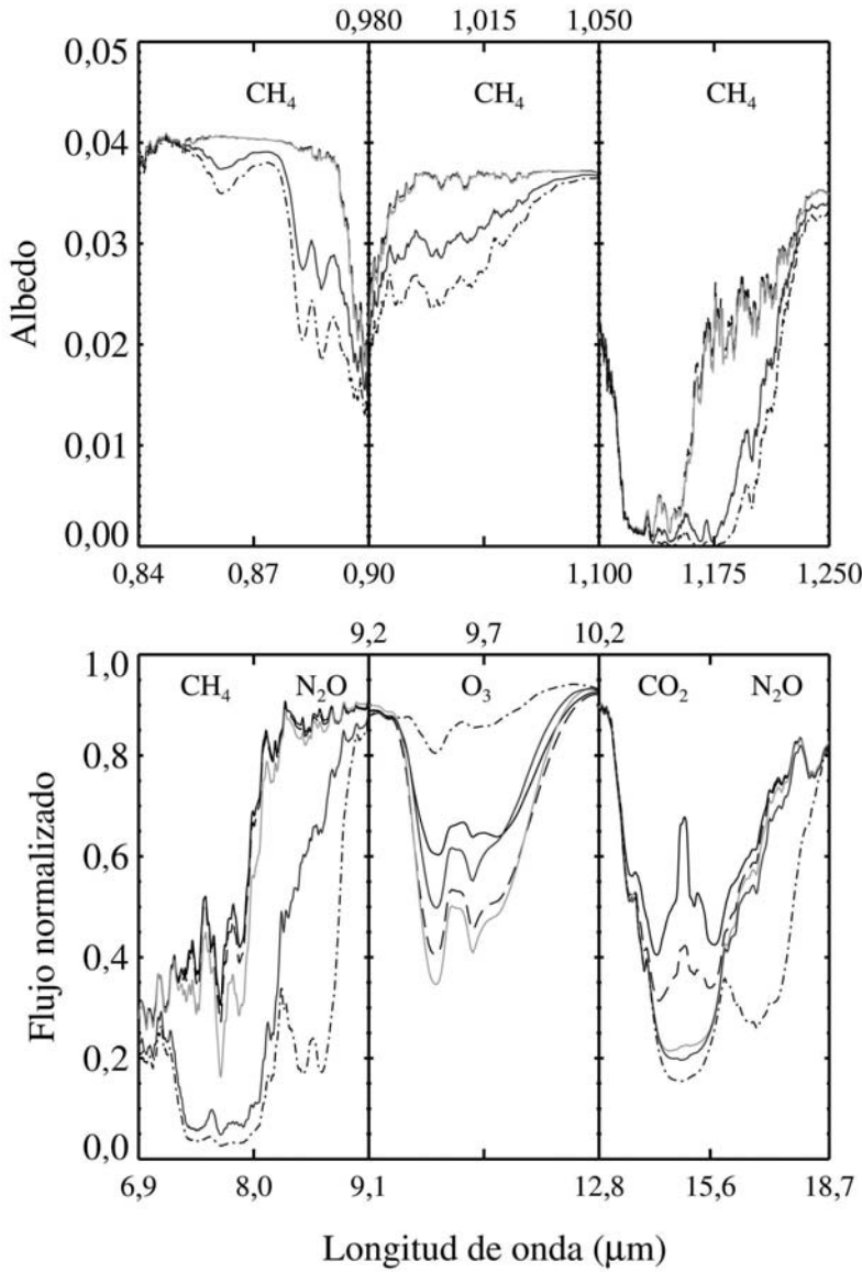
Fig. 5 - Bandas prominentes de CH 4 , N 2 O, O 3 , y CO 2 en el infrarrojo cercano (panel superior) y el infrarrojo medio (panel inferior) en espectros de planetas como la Tierra alrededor de estrellas F, G, K y M. El espectro en el infrarrojo medio está normalizado a un cuerpo negro con temperatura de 288 K. Clave: planeta alrededor de la estrella F: línea negra continua; planeta alrededor de la estrella G: línea negra discontinua; planeta alrededor de la estrella K: línea gris claro; planeta alrededor de la estrella M(AD Leo): línea gris oscuro; planeta alrededor de la estrella M(3100K): punto-rama negra. (Fuente: Segura et al. 2003 y 2005).
